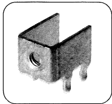
KP-18 (15A) 黄銅/半田メッキ 【M3、M4】
