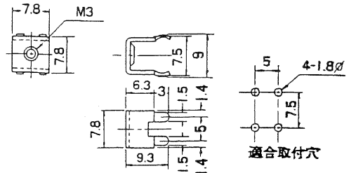
KP-19 (20A) 黄銅/半田メッキ 【M3】 (1t)
