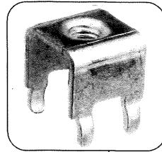
KP-17 (15A) 黄銅/半田メッキ 【M3、M4】
